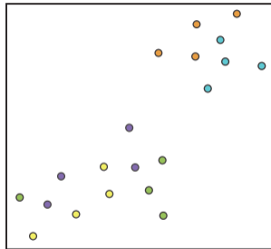
t-SNE
